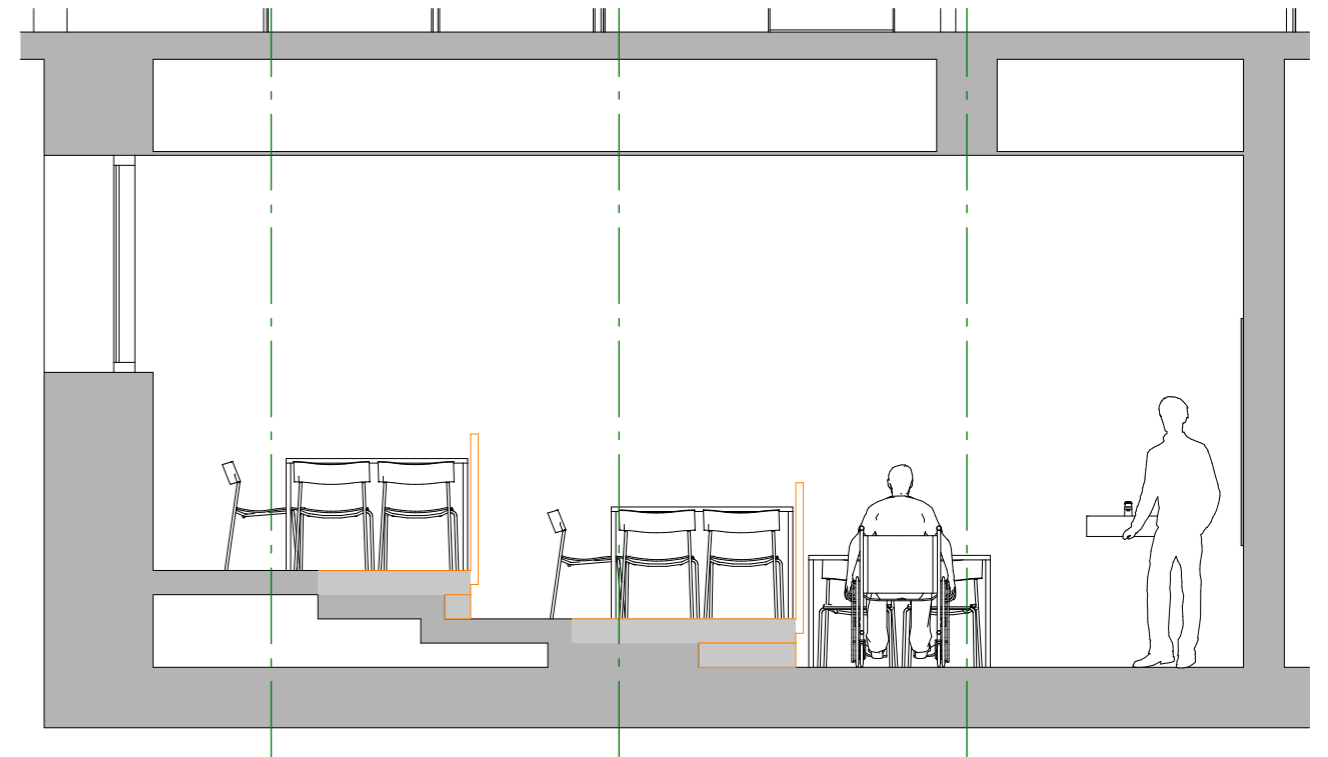
Snitt A-A
